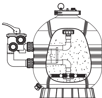
TYPISCHE INSTALLATION
